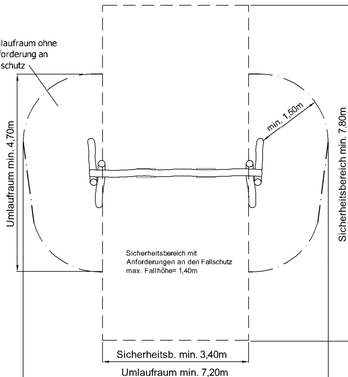
Doppelschaukel Robinie Art.-Nr.: 02 2927
