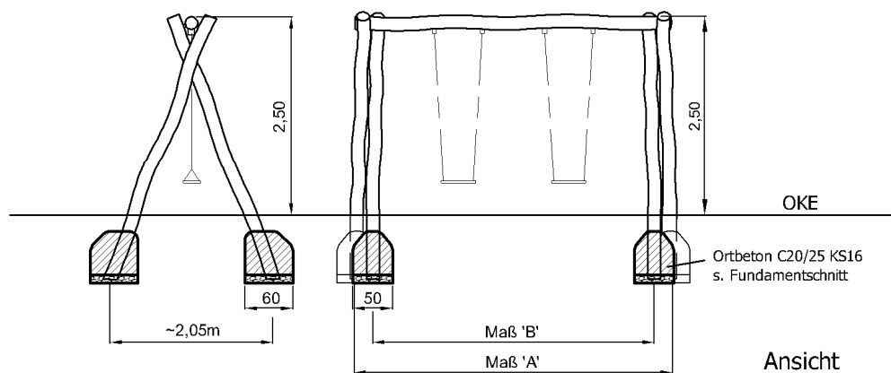
Doppelschaukel Robinie Art.-Nr.: 02 2927
