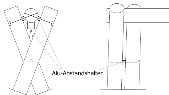
Anordnung Alu-Abstandshalter
