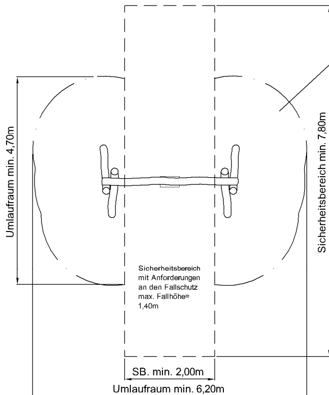
Einfachschaukel Robinie Art.-Nr.: 02 2926
